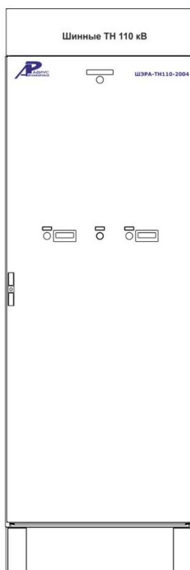
Шкаф шинных ТН 6-35 кВ ШЭРА-ТН110-2004 БПВА.656457.455, БПВА.650645.001 ТУ
